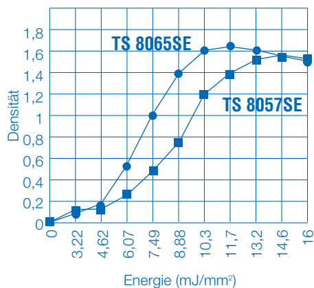
Dynamische Druckdichte 1454 Ohm, Atlantek 400
